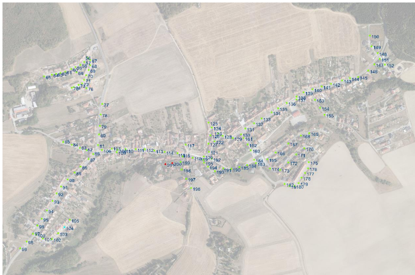
Obrázek 6: Technický stav svítidel (zelený – 1, modrý -2, červený – 3)
