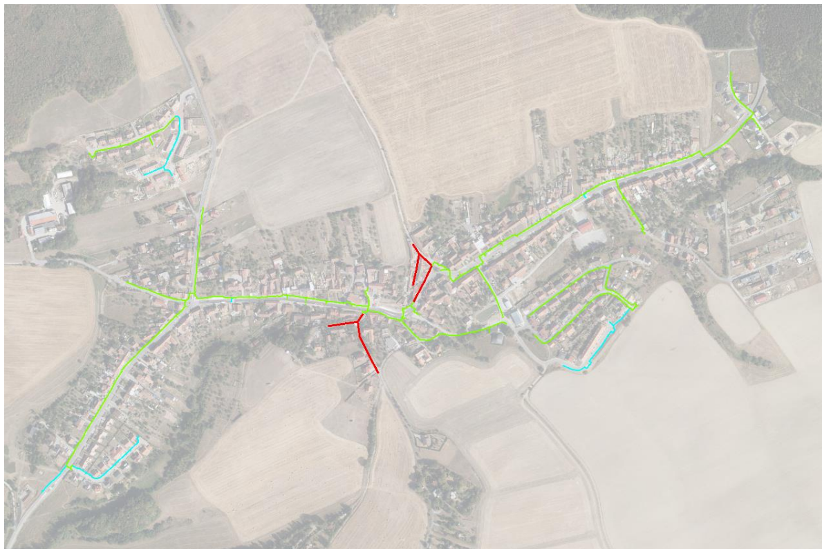
Obrázek 5: Uložení vedení VO (červená – nadzemní, zelená – zemní, zaměřené, modrá – zemní, orientační)
